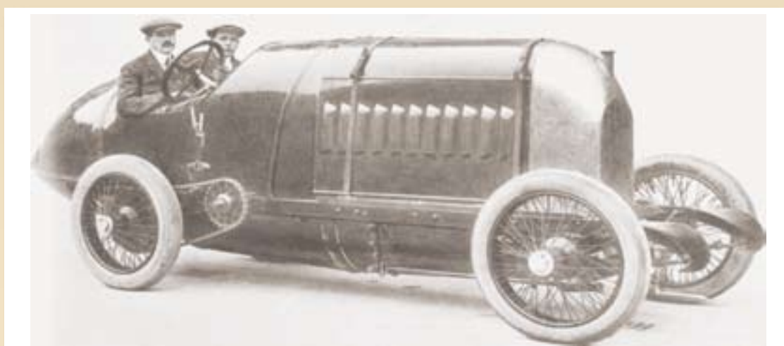
Fiat S.76 : un cofano monumentale per un motore gigante! L'auto fu esclusivamente prodotta per sfidare i record di Blitzen-Benz su una pista dritta. Sebbene avesse raggiunto a Ostenda una performance molto simile, non fu mai omologata. Da notare sulla parte anteriore, sotto il radiatore a forma di pera, l'aerodinamico becco d'aquila: fu questa una caratteristica disegnata per ridurre il 'valore Cx'?
